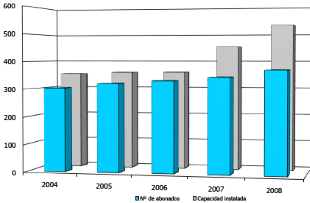
CAPACIDAD INSTALADA Y NÚMERO DE ABONADOS TELEFÓNICOS (en miles). PERIODO 2004-2008
